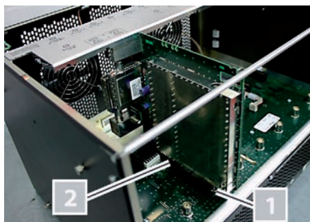
Bild 4a: Einbauzustand der Steckkarte (V 16 Basiseinheit)
