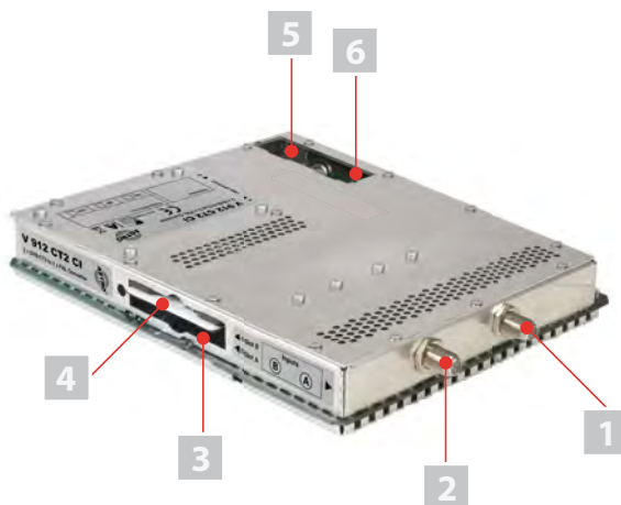
Bild 1: Steckkarte V 912 CT2 CI
