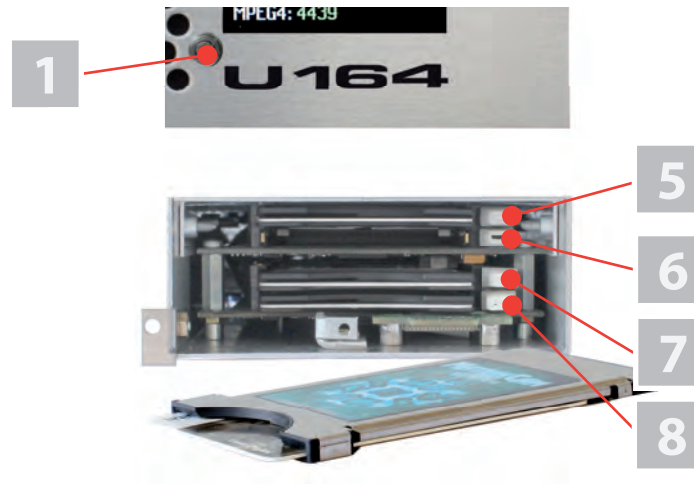
Bild 4: CI-Einschübe
