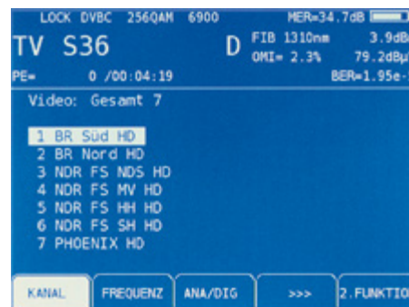
Messung eines optischen BK-Signals mit Auswertung der gewohnten HF-Parameter.
