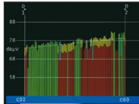
TILT-Messung: automatische Erkennung der QAM-Ordnung und Kompensation der Pegelabsenkung.
